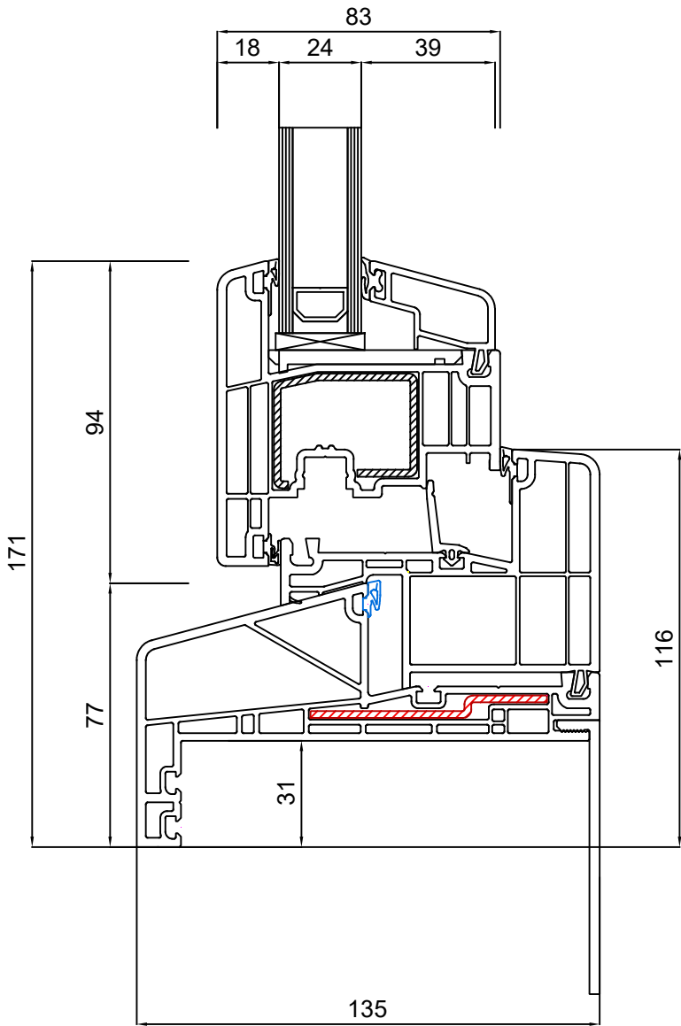
Detail: R2-B03-OD Schaal 1:2
